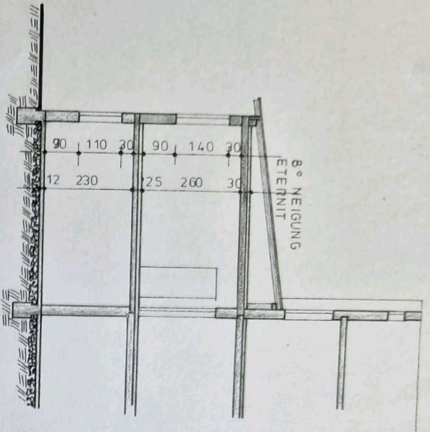
SCHNITTSCHEMA A-A
